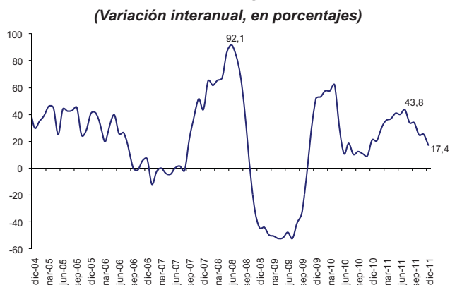
GRÁFICO II.15: ÍNDICE DE COTIZACIONES INTERNACIONALES DE ENERGÍA
