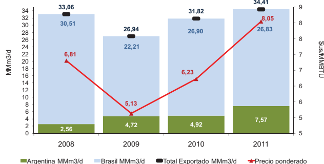
GRÁFICO III.3: VOLUMEN Y PRECIO PONDERADO 1/ DE EXPORTACIÓN DE GAS NATURAL AL MES DE DICIEMBRE DE CADA GESTIÓN (En MMm3/d y $us/MMBTU)
