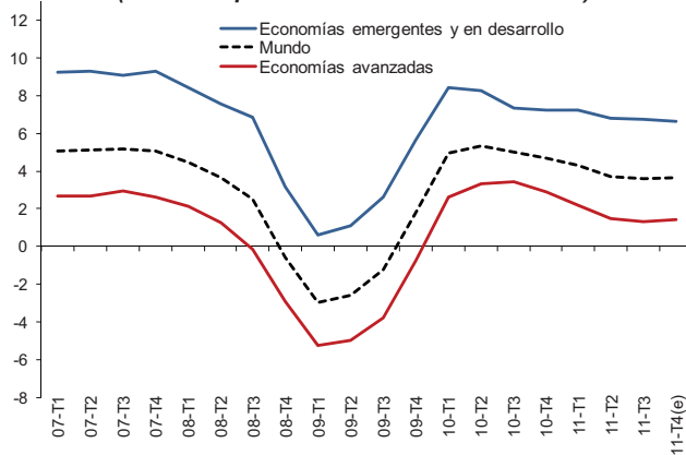
GRÁFICO I.1: CRECIMIENTO ECONÓMICO MUNDIAL (Variación porcentual trimestral interanual)
